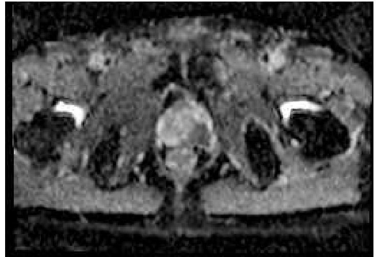
前立腺 ADCmap
