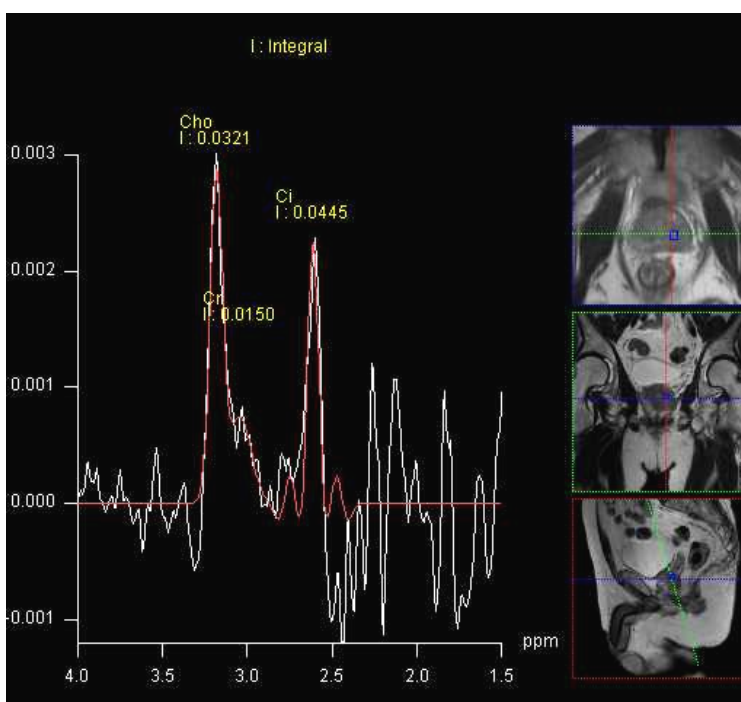
前立腺 MRS
